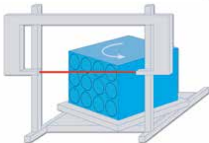
3. Materialauflagetisch dreht sich um 90°.
